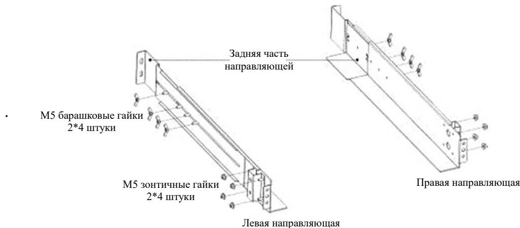
Рисунок 1 Сборка направляющих
