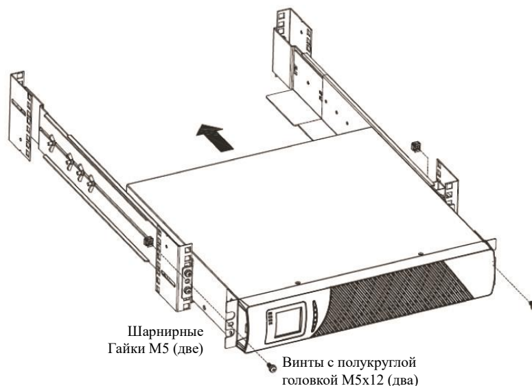
Рисунок 4 Крепление ИБП в шкафу спереди
