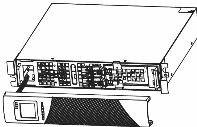
Рисунок 6 Подключение внутренних батарей ИБП
