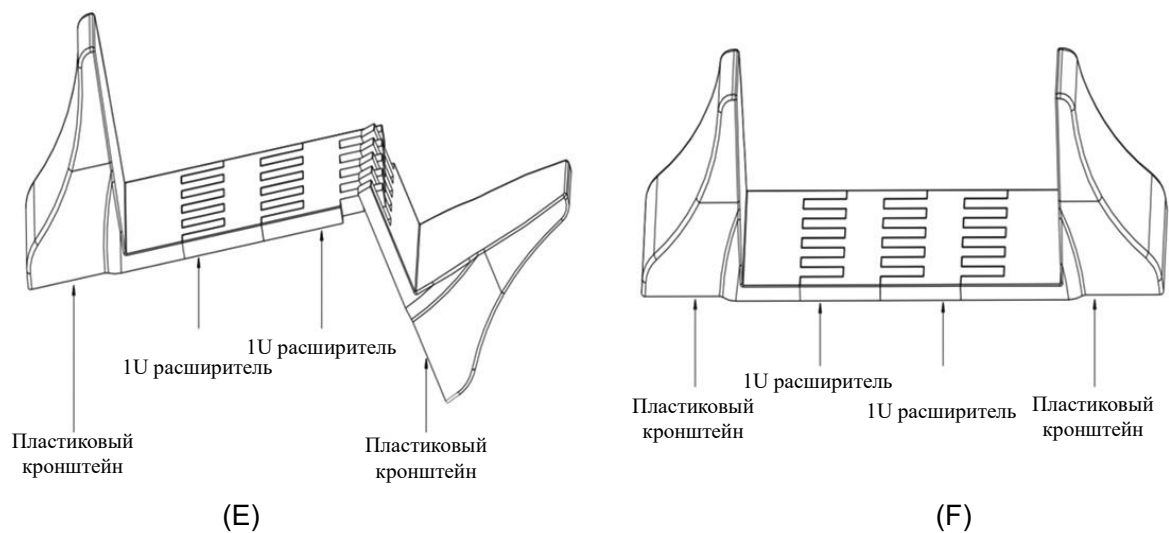
Рисунок 10 Расширение базы подставки
