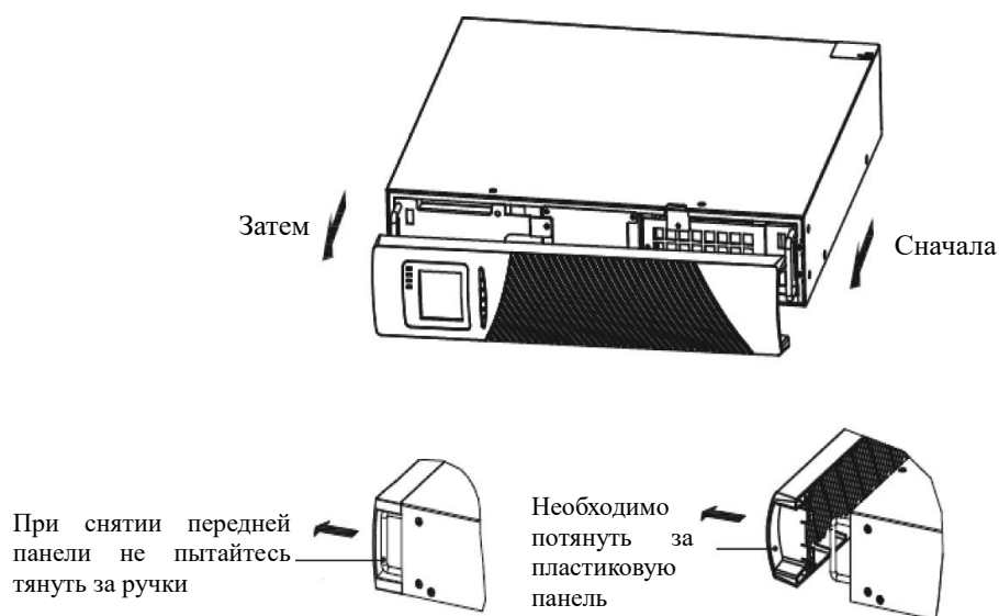
Рисунок 5 Снятие передней панели
