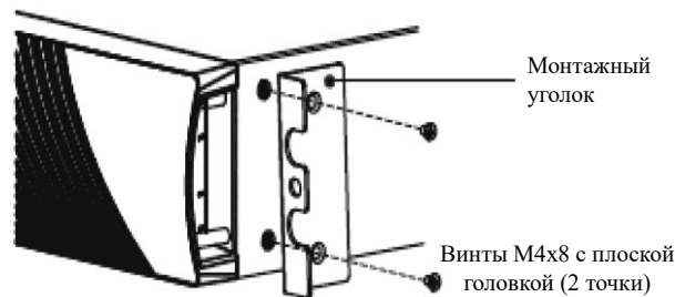
Рисунок 3 Установка монтажных кронштейнов
