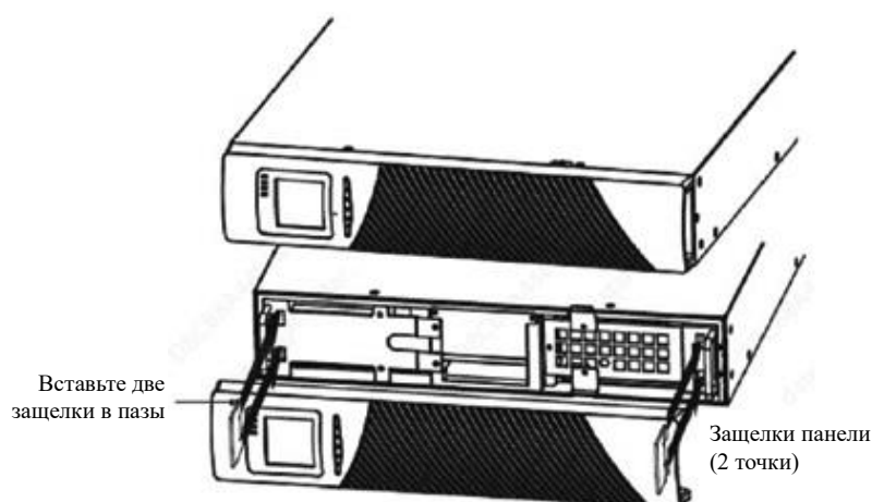
Рисунок 7 Установка лицевой панели
