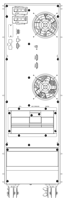
Вид сзади
