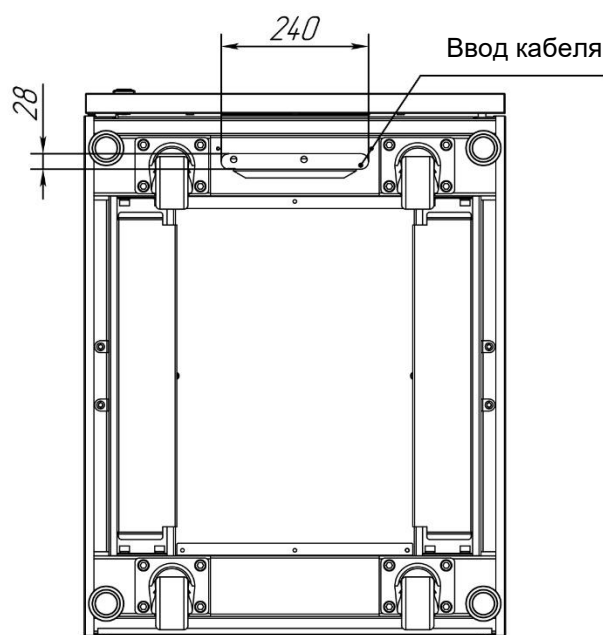
Вид снизу
